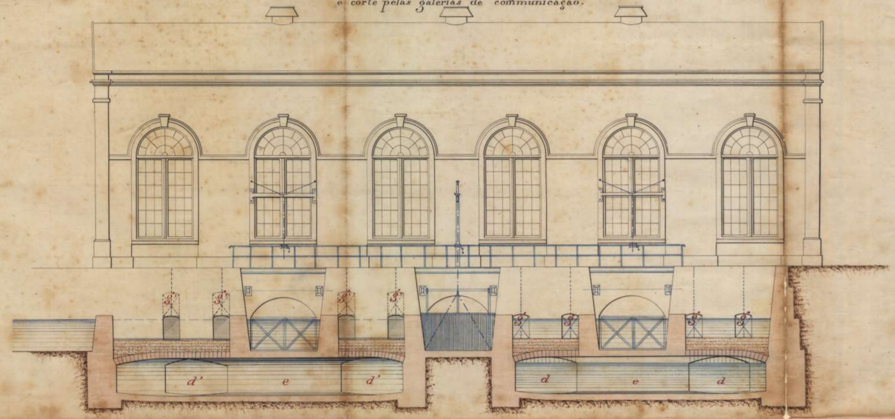
Corte transversal pelos filtros.
