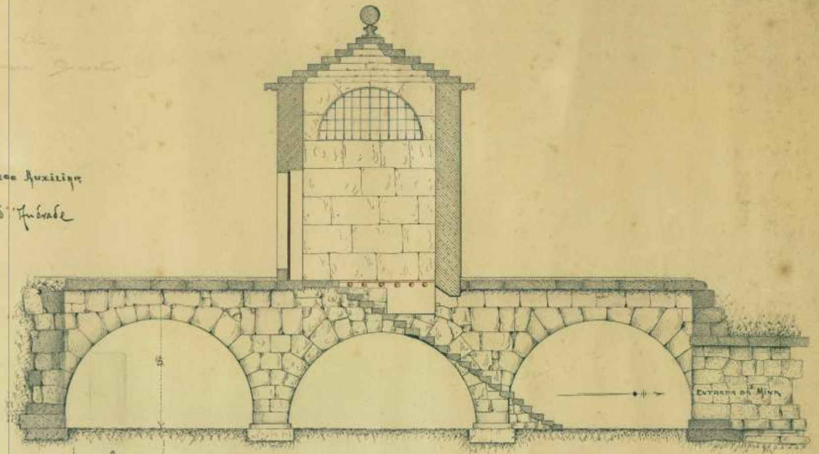
CORTE EM CD.
